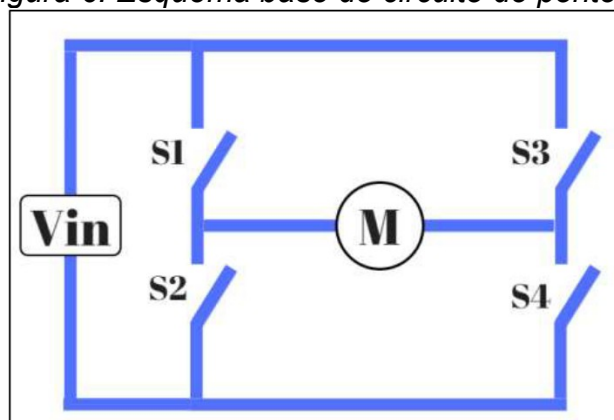
Figura 6: Esquema base do circuito de ponte h.
