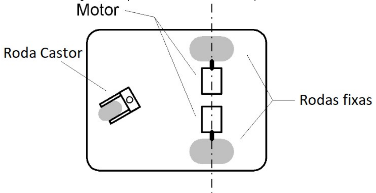
Figura 3: Esquema da estrutura do robô tipo uniciclo.
