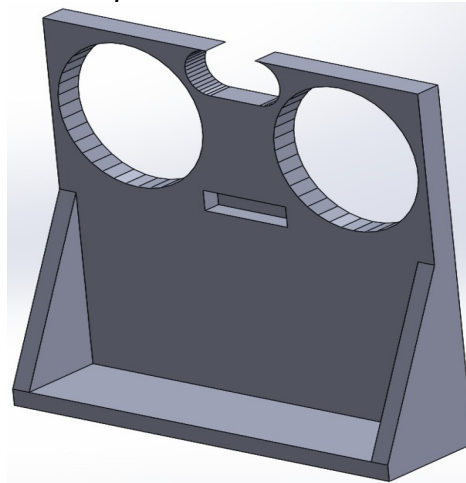
Figura 32: Ilustração em perspectiva do modelo mecânico do suporte frontal para o sensor HC-SR04.
