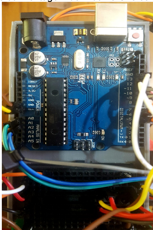
Figura 42: Foto da montagem do Arduino Uno com o protoboard.
