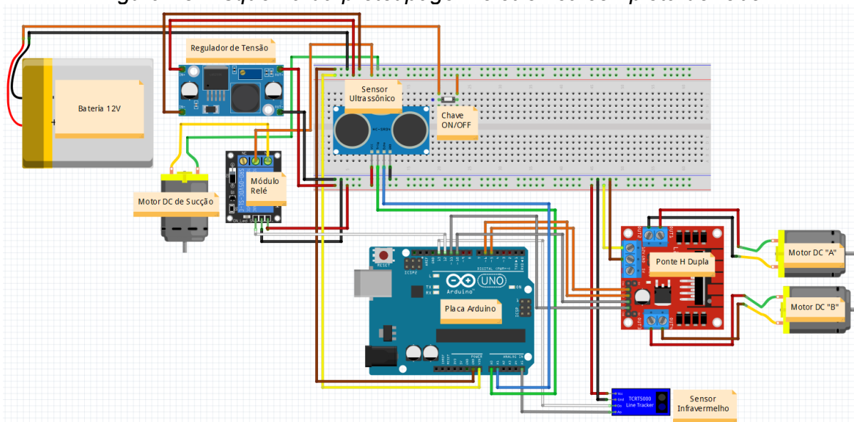
Figura 28: Esquema da prototipagem eletrônica completa do robô.
