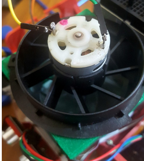
Figura 45: Foto da montagem do motor de sucção.
