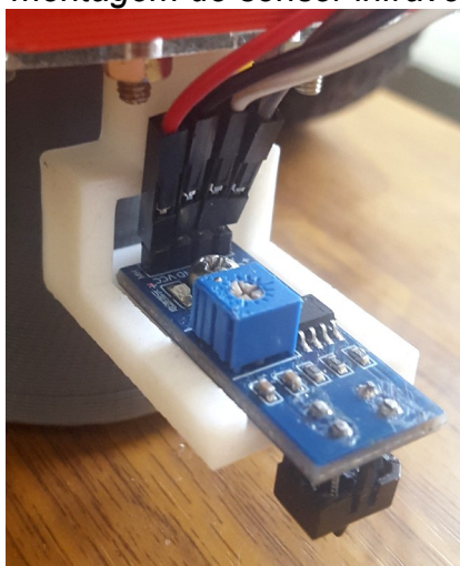
Figura 41: Foto da montagem do sensor infravermelho TCRT5000.
