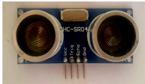
Figura 18: Foto do módulo sensor ultrassônico HC-SR04.
