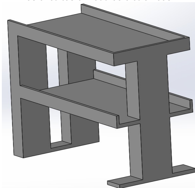
Figura 39: Ilustração em perspectiva do modelo mecânico do suporte para os circuitos e módulos eletrônicos.
