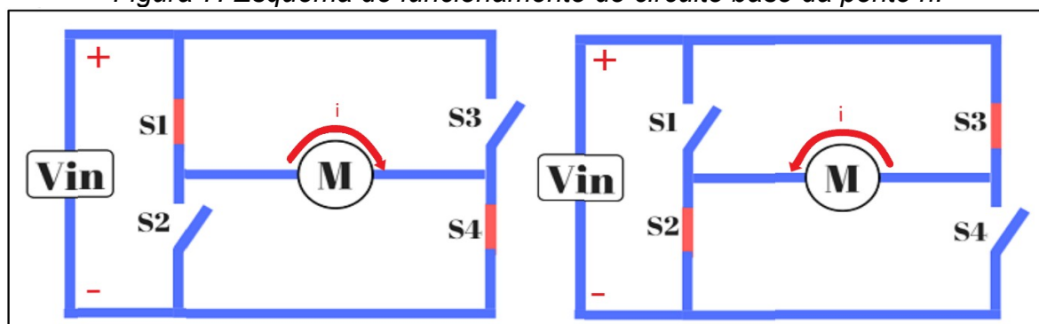
Figura 7: Esquema de funcionamento do circuito base da ponte h.
